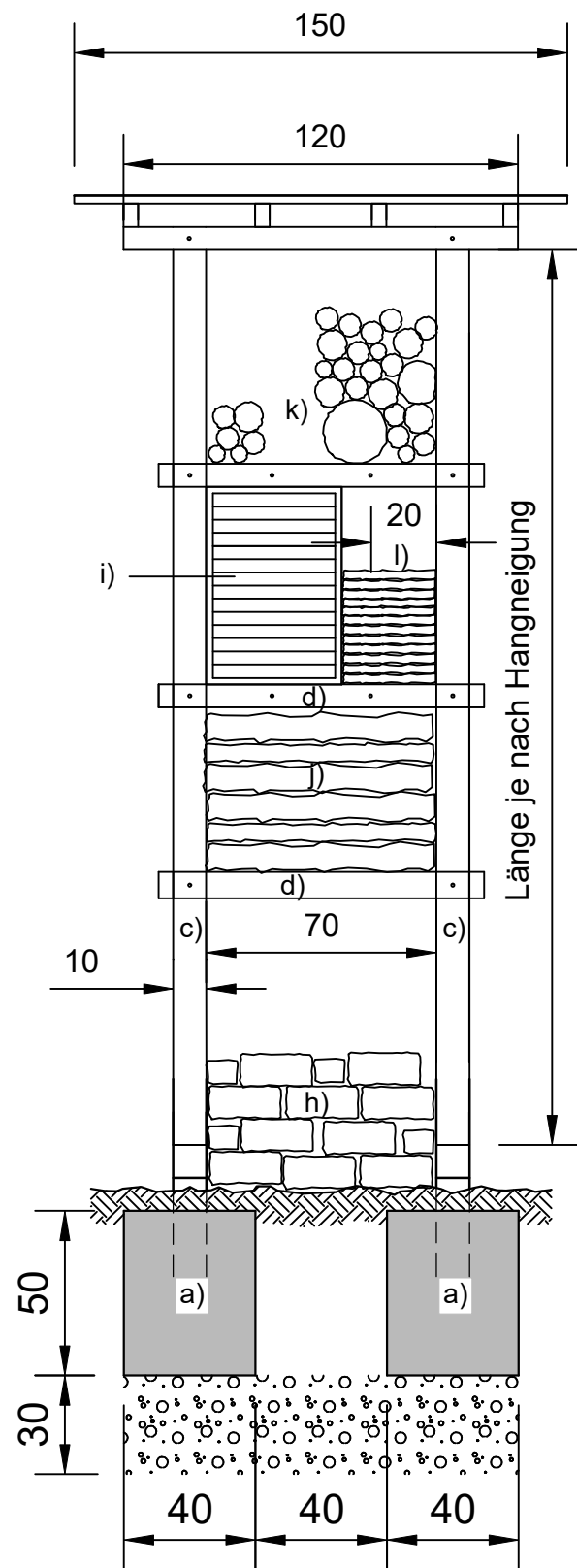
Frontansicht
